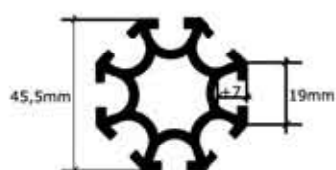
Perfil
